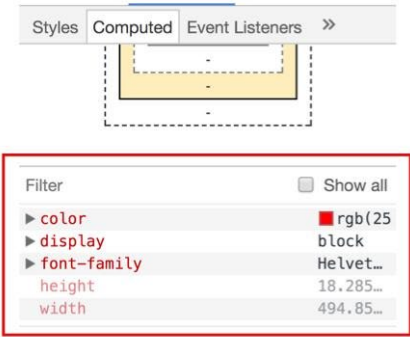
Chrome Devtools (narrow width)
